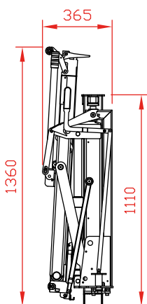
OWU006 in rijpositie rechts gemonteerd
