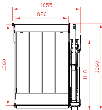
OWU006 in werkpositie rechts gemonteerd
