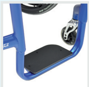
Gelaste aluminium voetsteun met kunststof plaat
