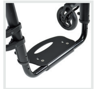
Eendelige aluminium voetplaat met gebogen buizen, in hoogte en hoek verstelbaar
