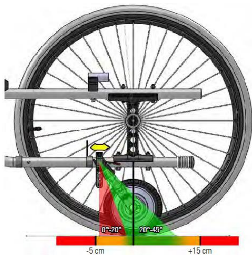
Montage Breezy X-Family rolstoelen met Empulse R20
